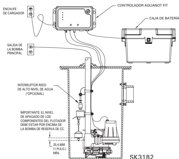
BOMBA DE CC INSTALADA EN LÍNEA CON BOMBA SUMERGIBLE
